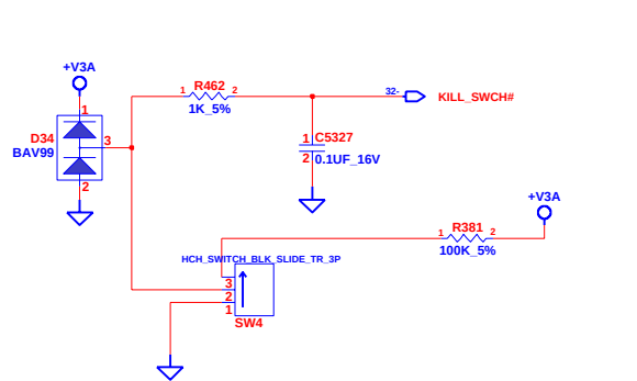
KILL SWITCH
