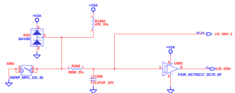
LID SWITCH
